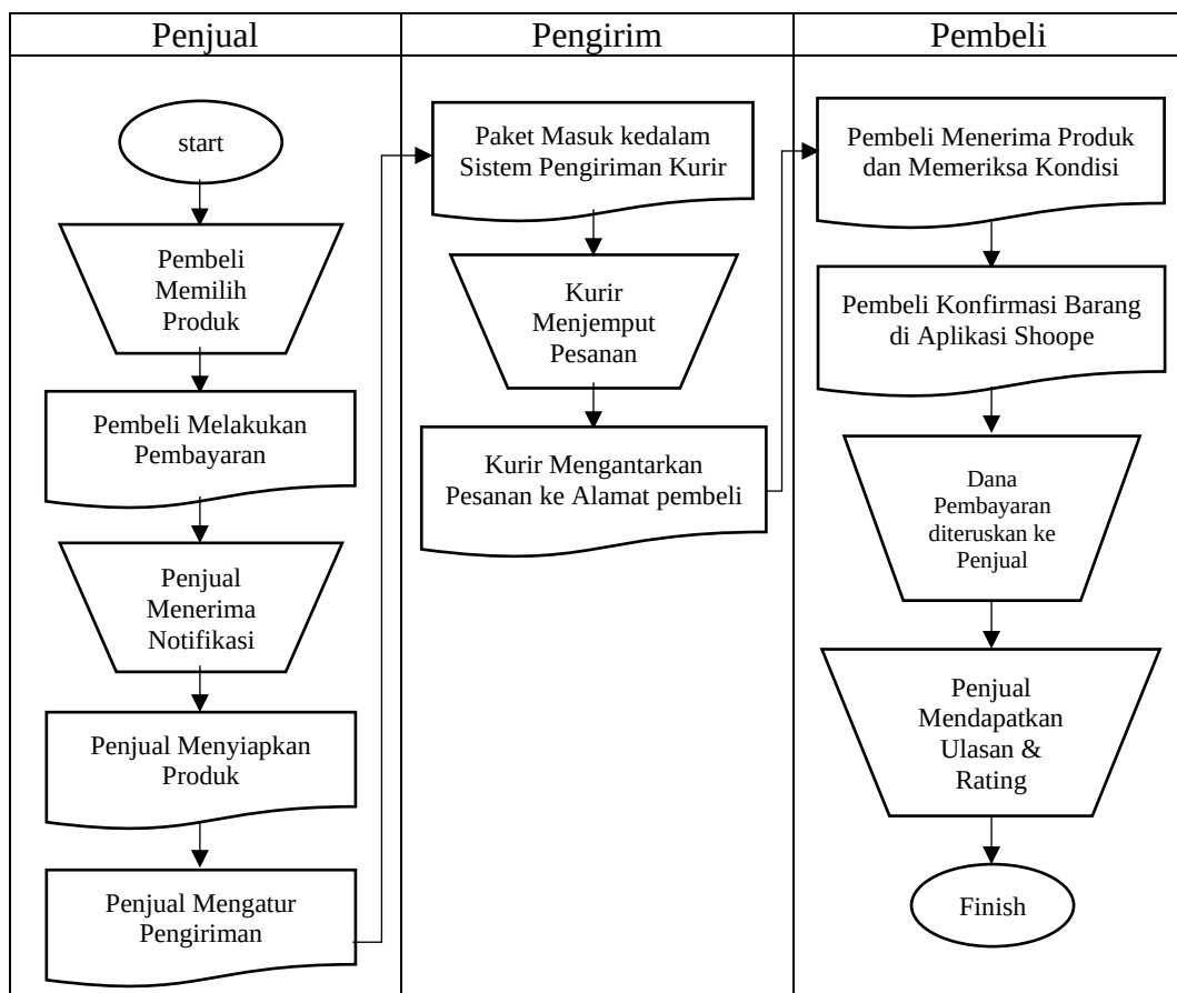
Gambar 3. Flowchart Usulan Penjualan (pelanggan melalui aplikasi Shoope)
